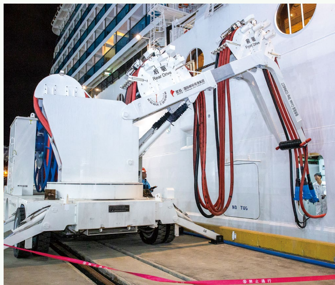
➤ 厦门国际邮轮母港邮轮泊位岸电系统
